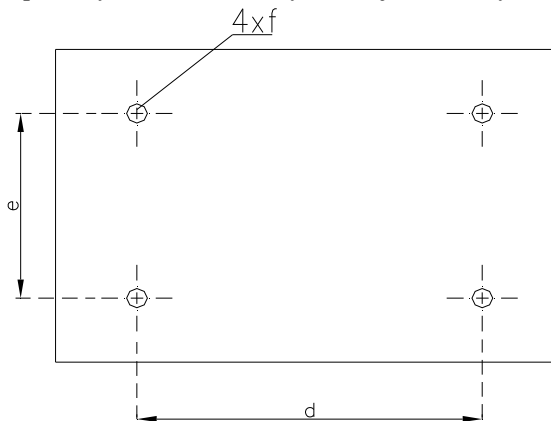
Widok "W" Rozmieszczenie otworów mocujących
