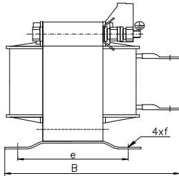
Wykonanie z końcówkami kablowymi
