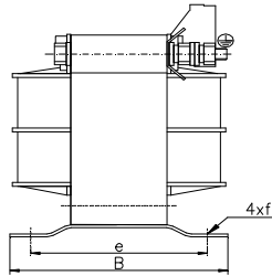
Wykonanie z zaciskami śrubowymi
